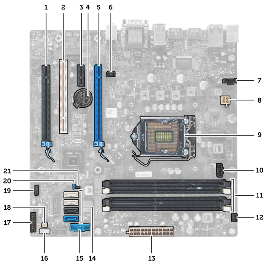
Kuva 1. Emolevyn komponentit
